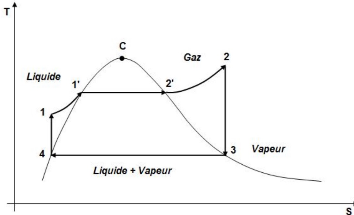
Figure 6. Le cycle de Hirn sur diagramme (T, S)
