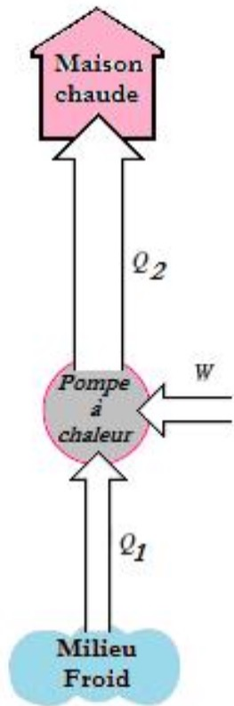
Fig. 5.13. Machines dynamo-thermiques (Pompe à chaleur)
