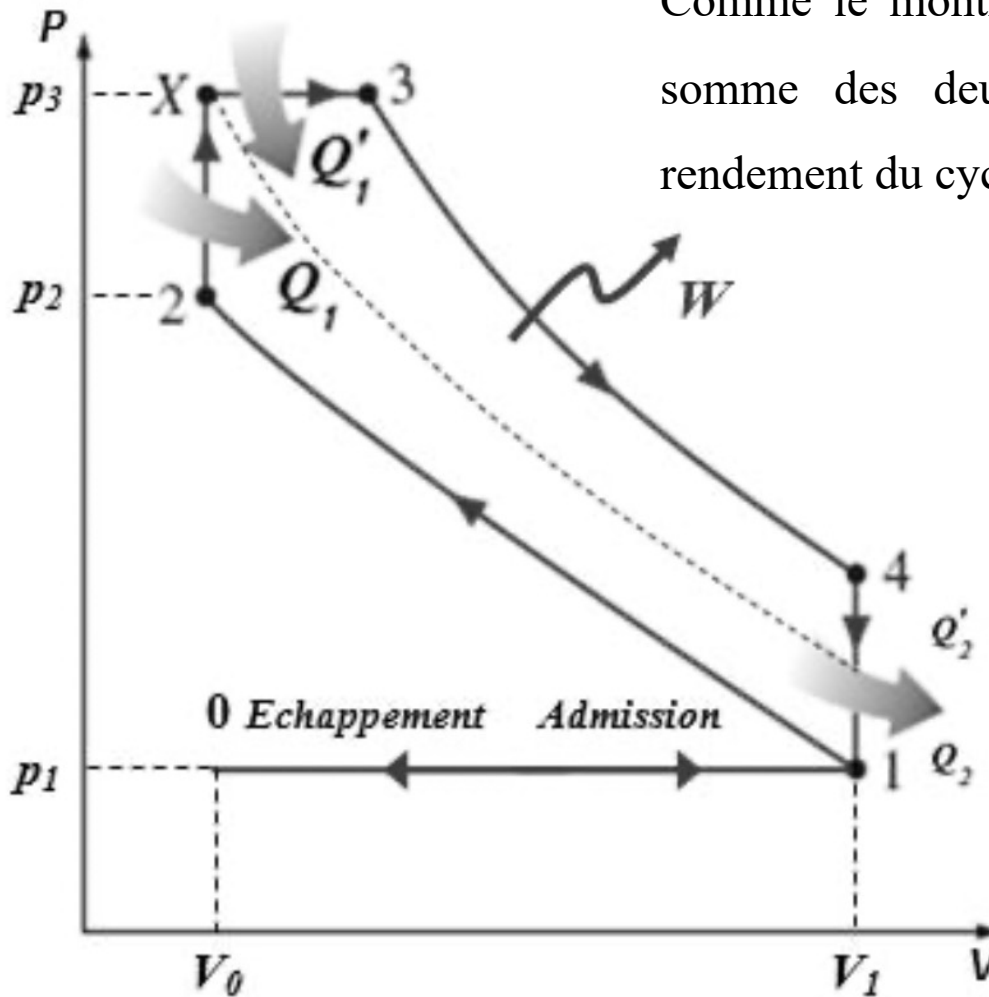
Figure 5.8. Cycle de Sabathé (cycle mixte)
