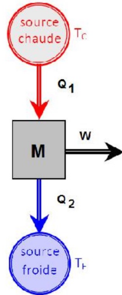
Figure 1. Schéma de principe d'une machine dithermes motrice
