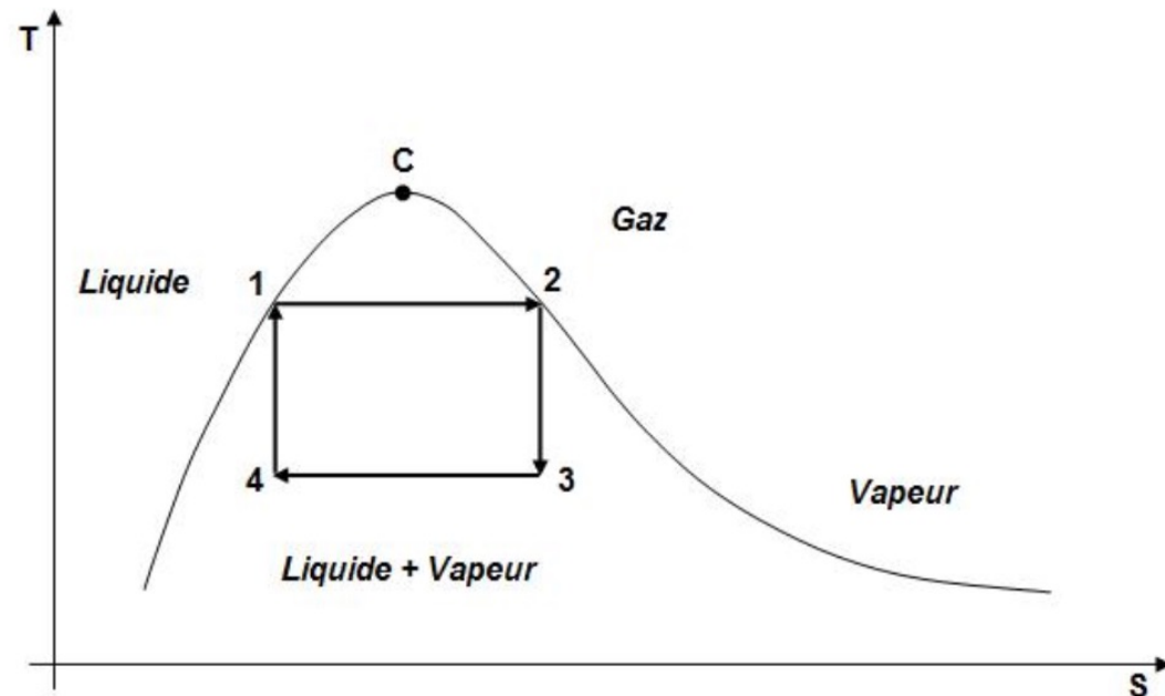
Figure 4. Représentation du cycle de Carnot sur un diagramme ( T, S )
