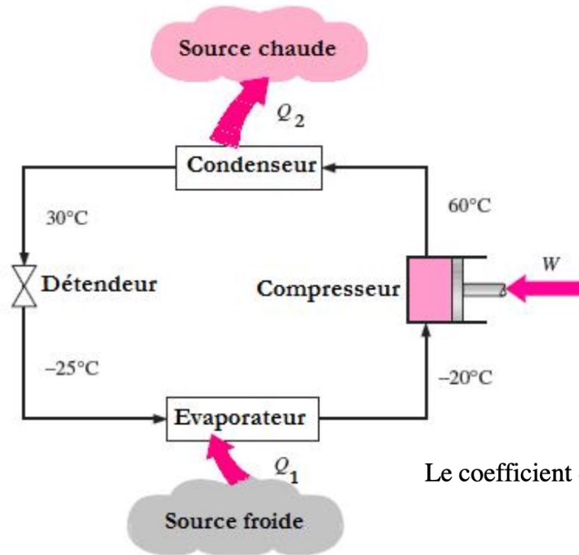
Fig. 5.12. Machines dynamo-thermiques (Réfrigérateur)
