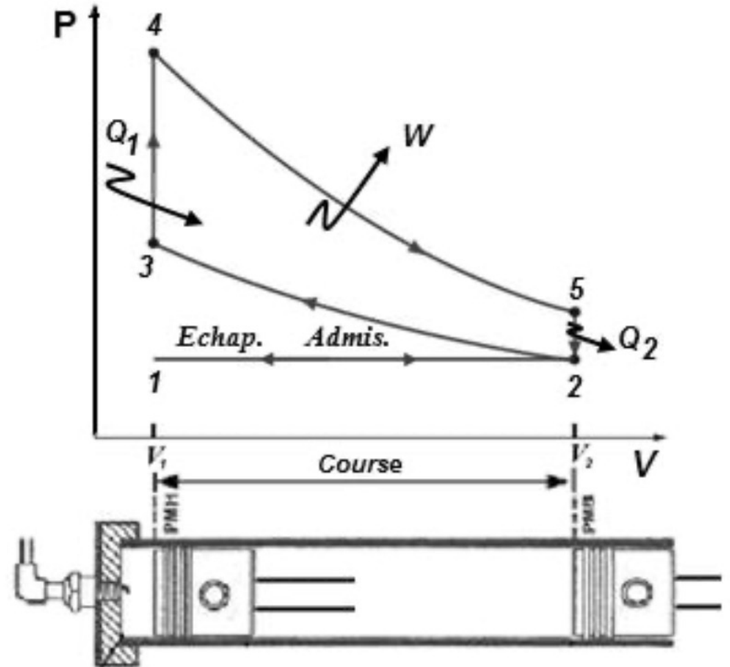
Figure 5.6. Cycle de Beau de Rochas
