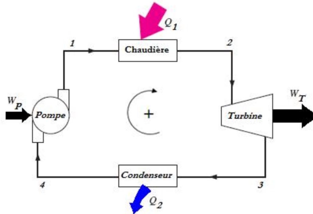
Figure 2. Schéma de principe d'une machine thermique motrice à cycle fermé (Moteur à vapeur)
