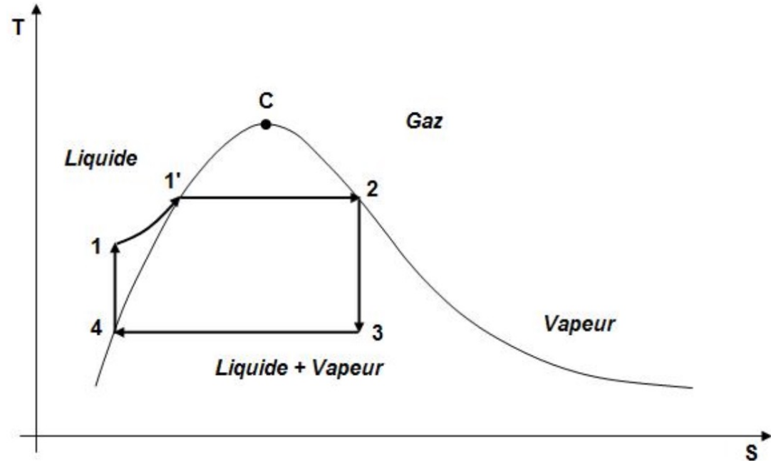
Figure 5. Le cycle de Rankine sur diagramme (T, S)
